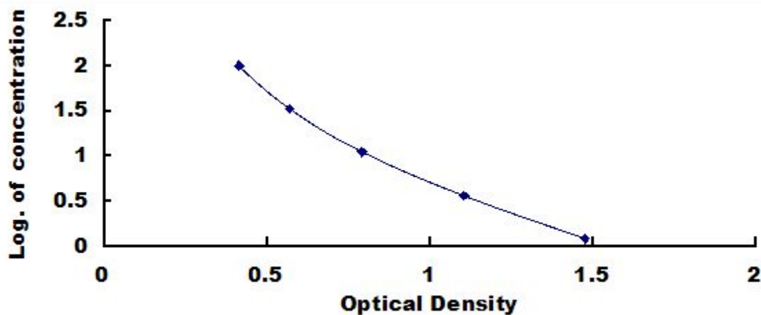
谷胱甘肽 (GSH) 检测试剂盒标准曲线
