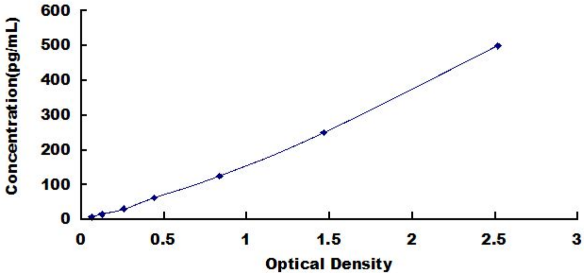
小鼠 cAMP 应答元件结合蛋白 (CREB) 检测试剂盒标准曲线
