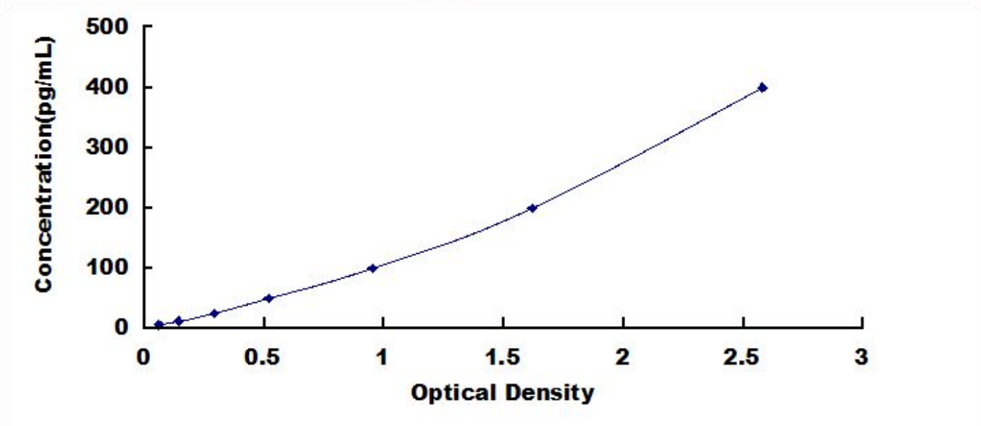
人白介素 6 (IL6) 检测试剂盒标准曲线
