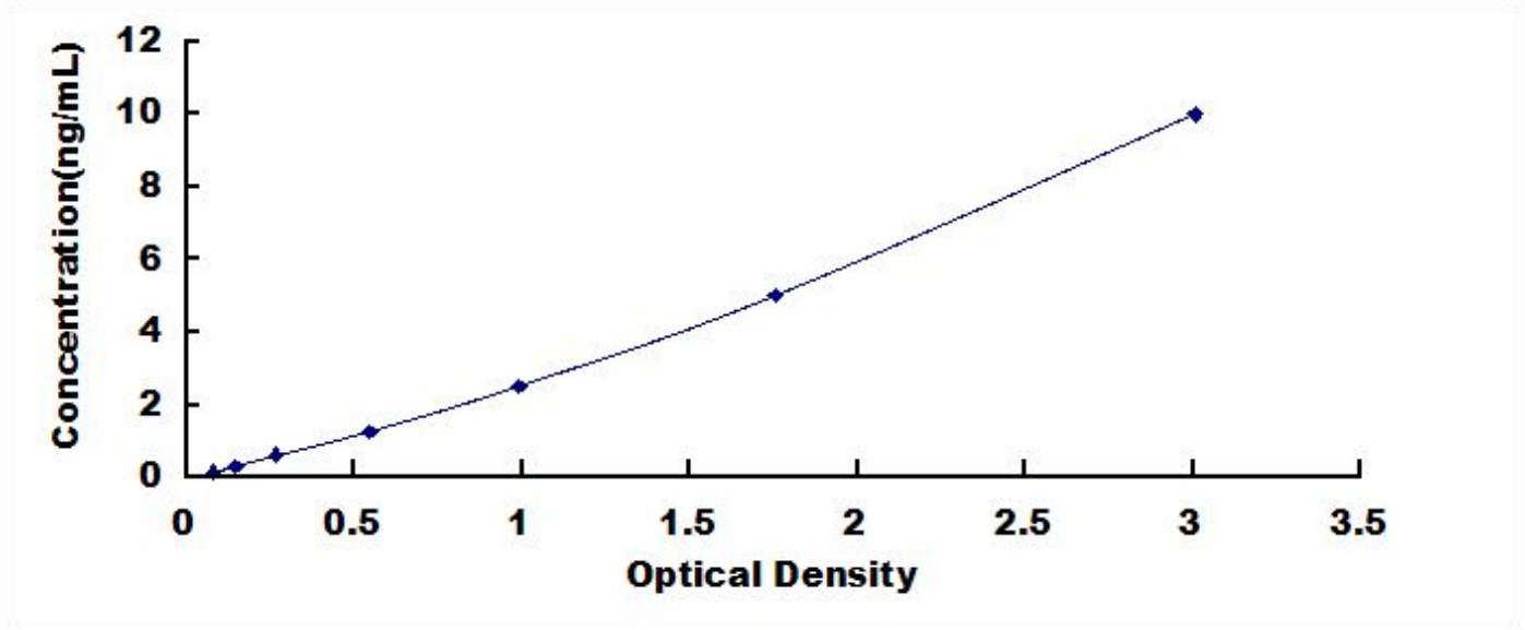
小鼠肿瘤坏死因子受体超家族成员 5 (CD40) 检测试剂盒标准曲线
