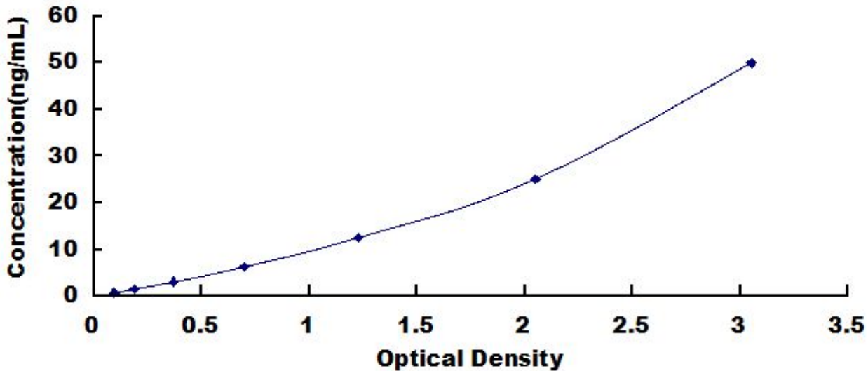
人钠/葡萄糖协同转运蛋白 2(SGLT2)检测试剂盒标准曲线
