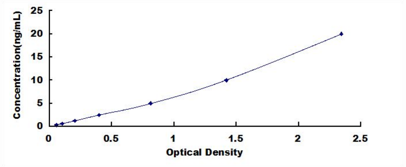
人蛋白精氨酸甲基转移酶 1 (PRMT1) 检测试剂盒标准曲线
