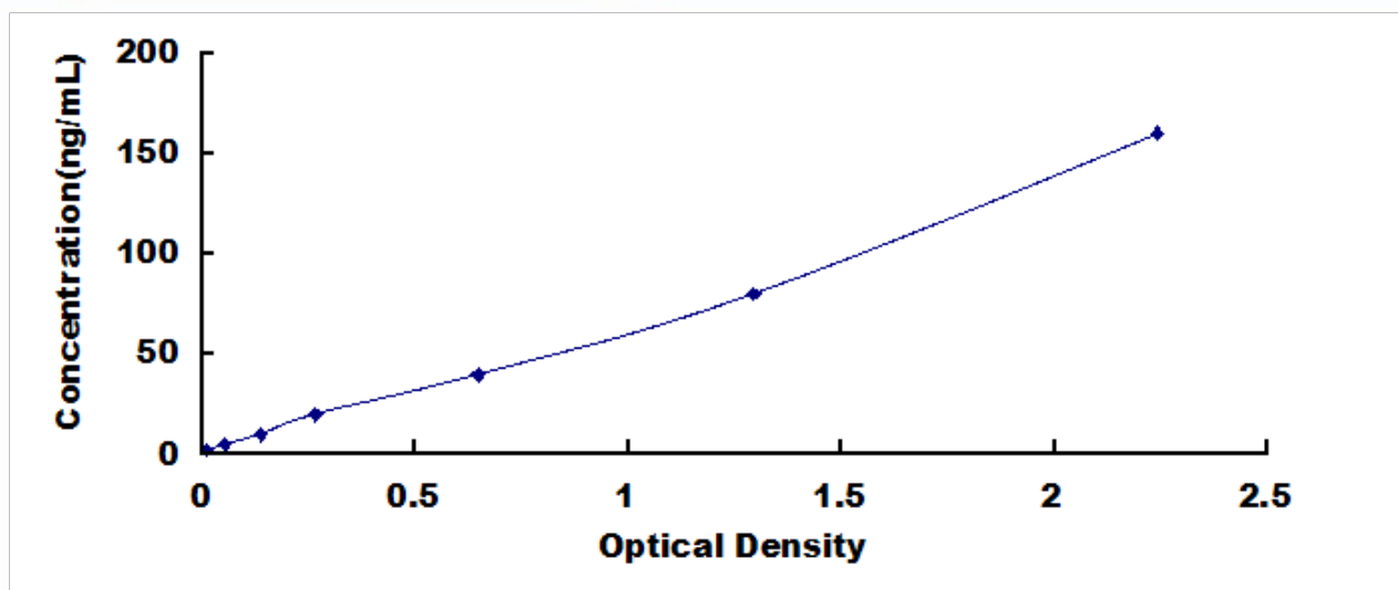
大鼠Ⅲ型前胶原 (PCIII) 检测试剂盒标准曲线
