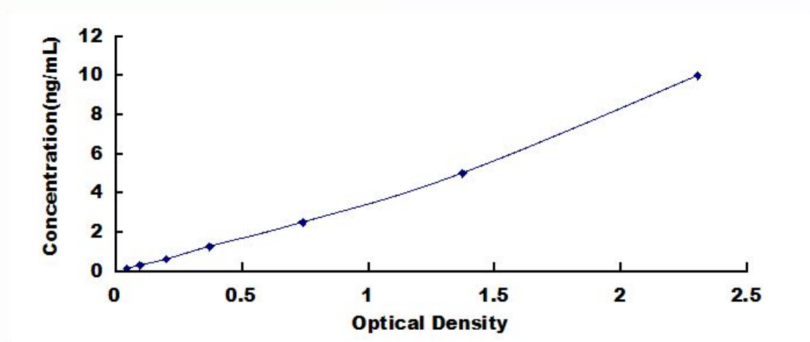
小鼠中性粒细胞弹性蛋白酶(ELA2)检测试剂盒标准曲线
