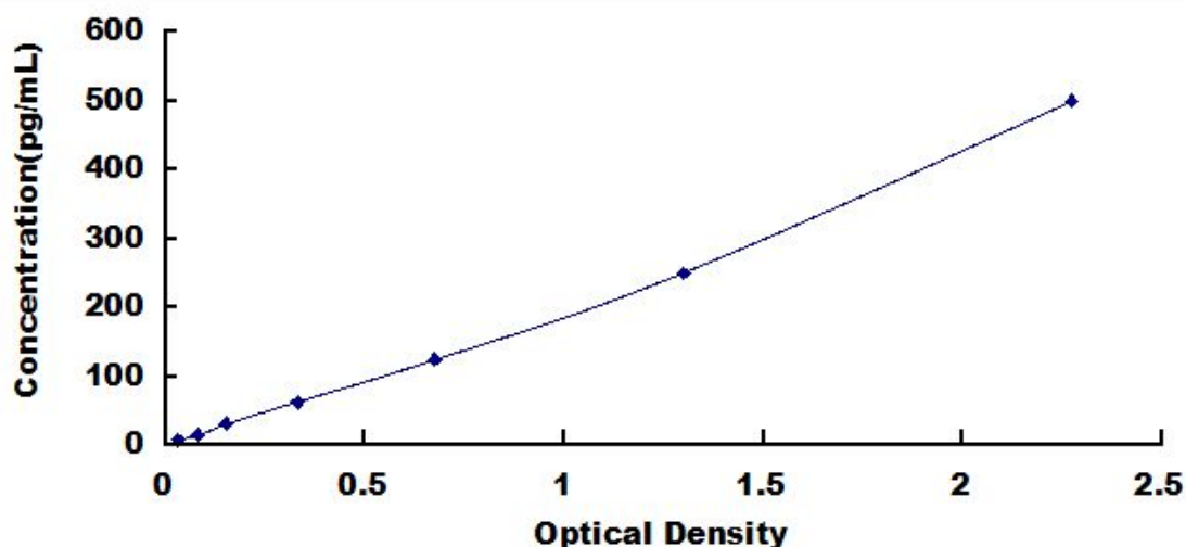
兔白介素 5 (IL5) 检测试剂盒标准曲线
