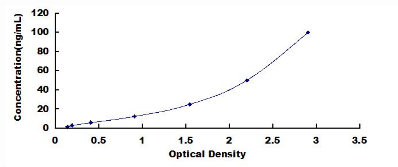
小鼠酪蛋白 α (CSN1)检测试剂盒标准曲线
