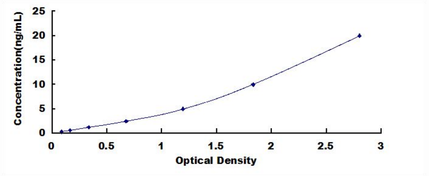
人酰基辅酶 A 脱氢酶 C4-C12 直链 (ACADM) 检测试剂盒标准曲线
